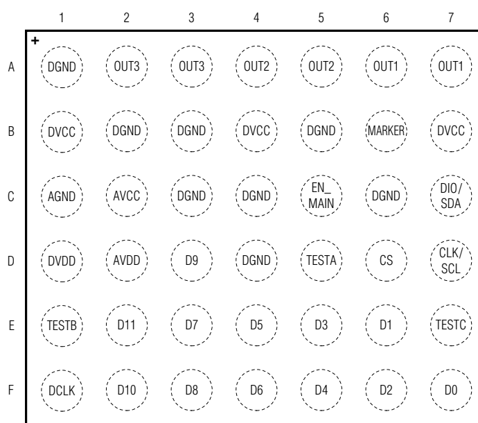
WLP (3.5mm x 3.0mm)
